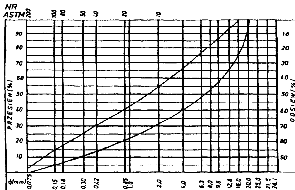
Rys. 2. Krzywe graniczne uziarnienia mieszanki mineralnej 0+20 mm do warstwy wiążącej z betonu asfaltowego dla KR 1-2
